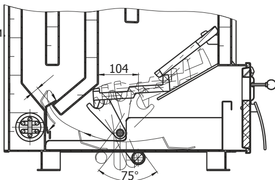
Рис.3 - Работа механизма перемещения колосника и установка заглушки прочистного отв.
